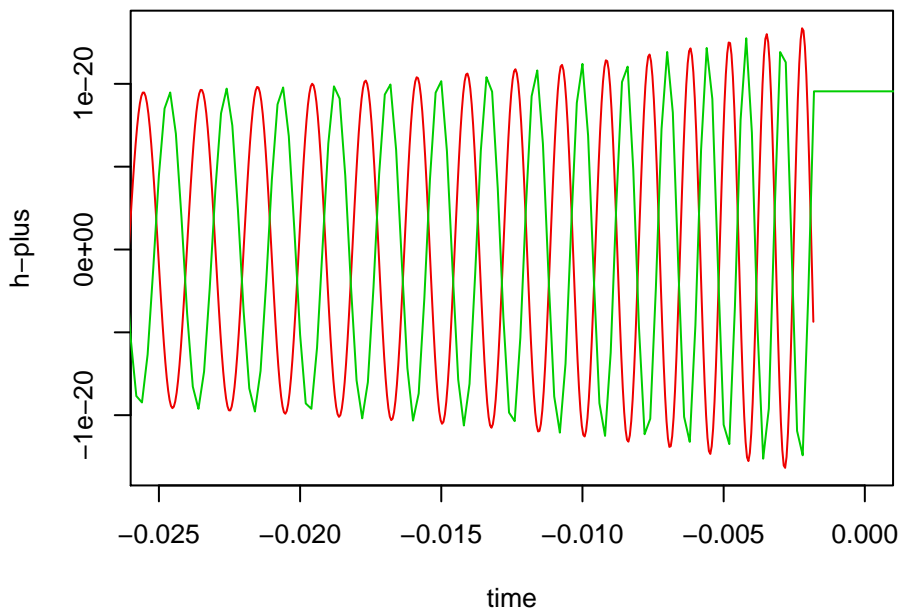
1.4 – 1.4 sun mass inspiral, \iota=0^\circ
