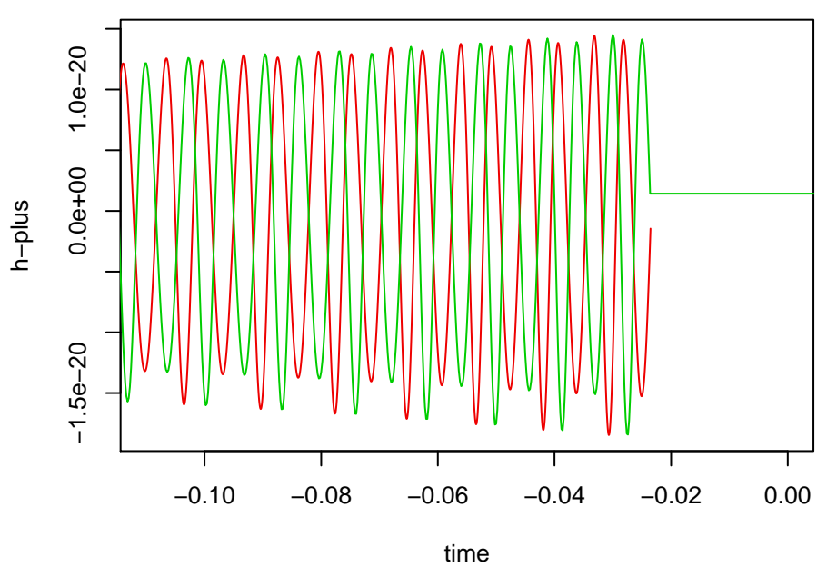
1.4 – 9.0 sun mass inspiral, \iota=45^\circ
