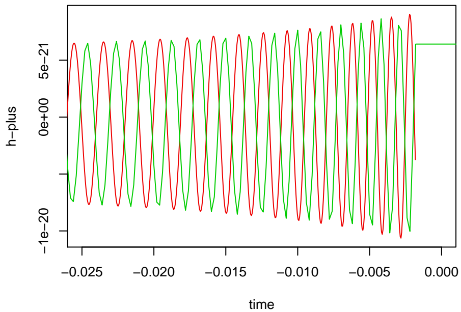
1.4 – 1.4 sun mass inspiral, \iota=45^\circ
