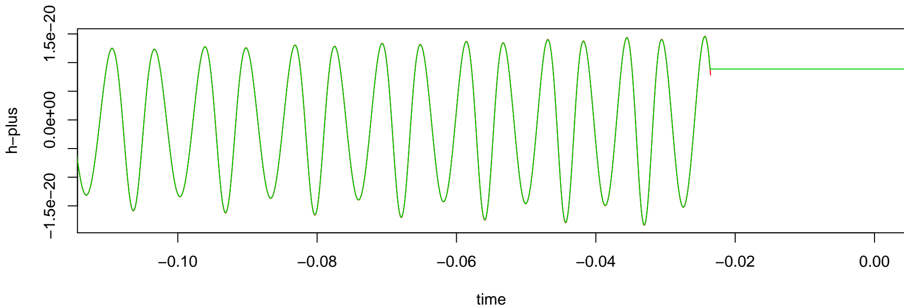
1.4 – 9.0 sun mass inspiral, \iota=45^\circ
