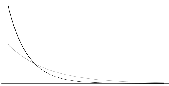
P.d.f., f_X(x)
