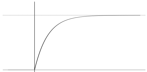
C.d.f., F_X(x) = \mathbb{P}(X \leq x) .
